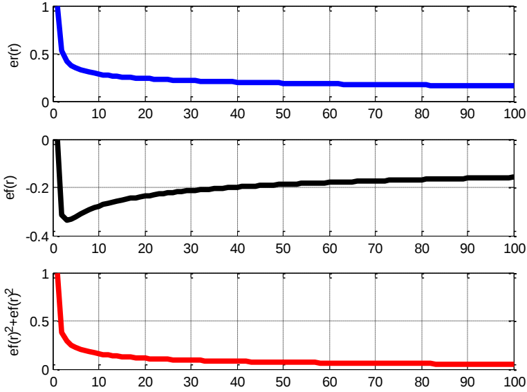
Fig.1. SecondSolMax.m
