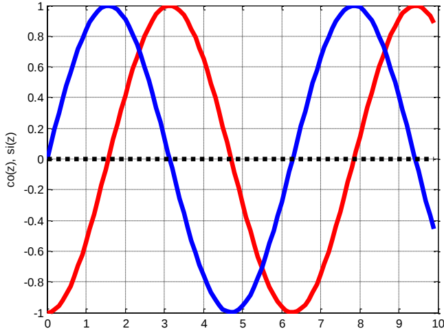
Fig.4. SecondSolMax.m
