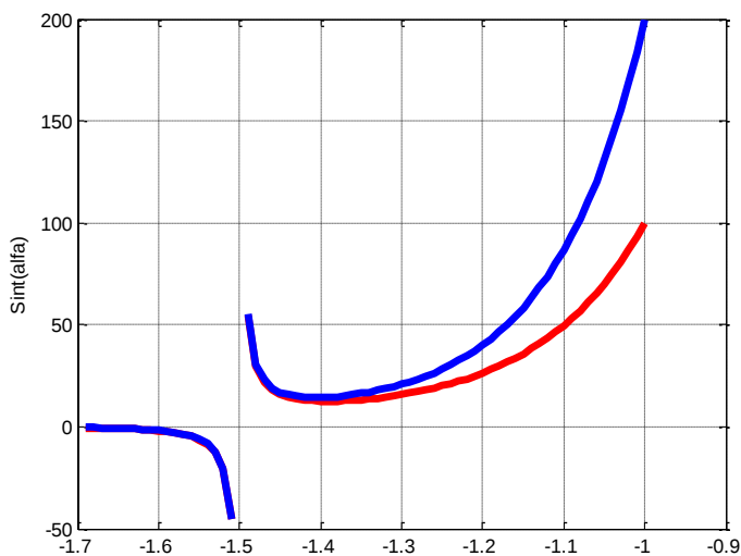
Fig.3. SecondSolMax.m
