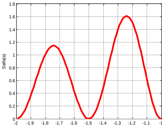
Fig.2. SecondSolMax.m
