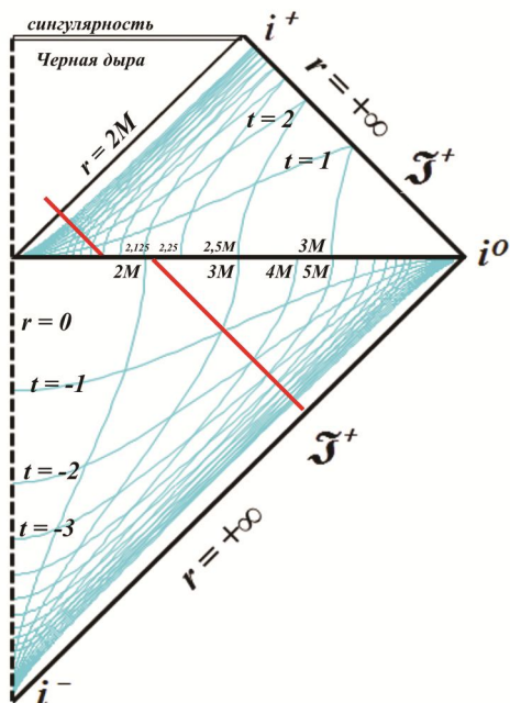
Рис.5.2. Диаграмма коллапсирующей нейтронной звезды с сеткой времени и расстояний. Нулевая геодезическая может быть изображена только ломаной линией.
