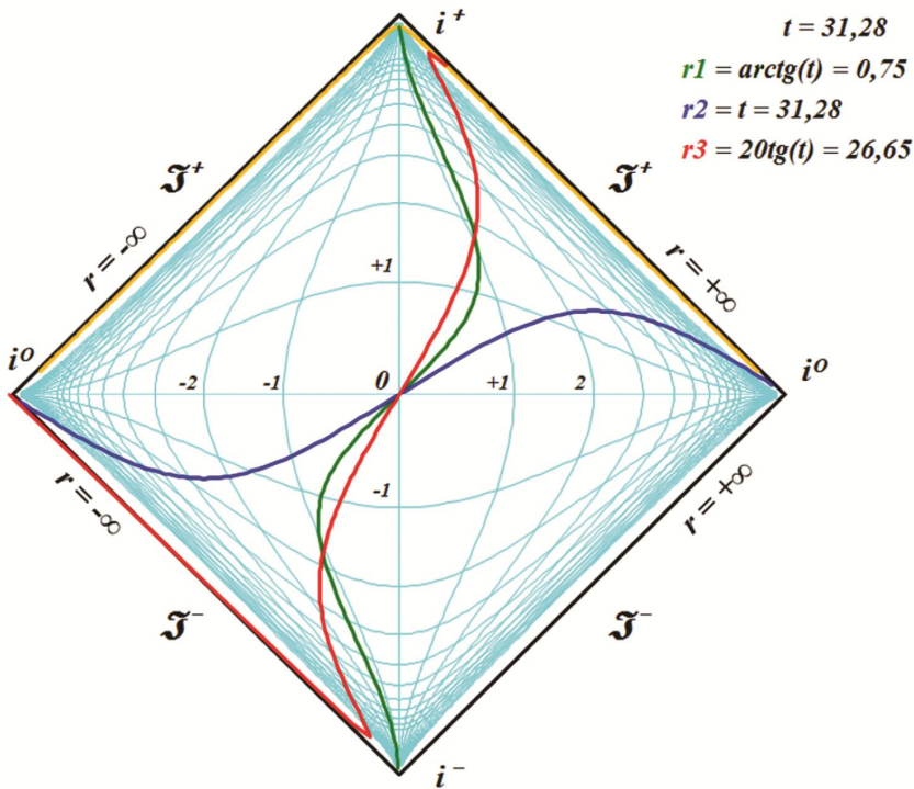
Рис.2.8. Попытки получить аналитическое уравнение прямой мировой линии
