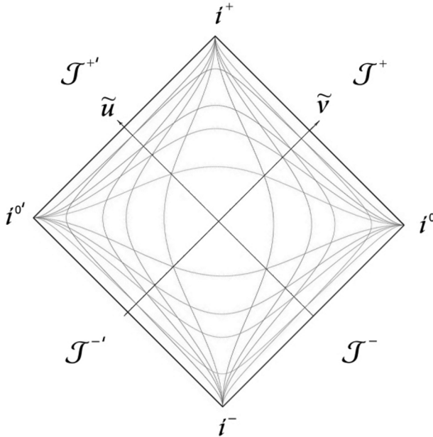
Рис.1.4. Исходная диаграмма Пенроуза [27]
