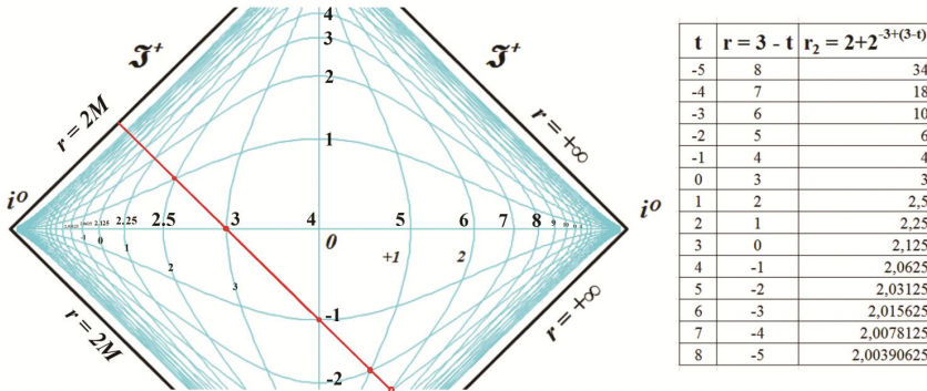
Рис.4.8. Диаграмма Пенроуза для вечной Черной дыры
