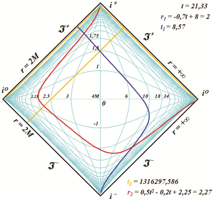
Рис.4.15. Мировые линии космолетов, движущихся к Черной дыре. Кадр из анимации [6]
