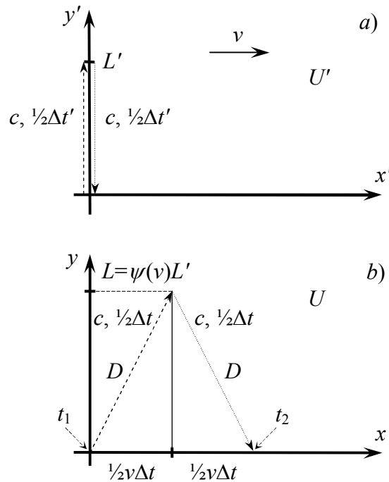
Рис. 2. Путь, проходимый светом, видимый из двух систем отсчета. а) инерциальная система отсчета U' , б) универсальная система отсчета U .
