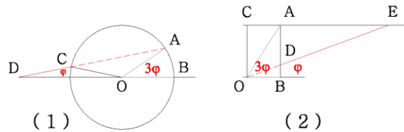
F.8. → (1) Archimedes , (2) Pappus Method
